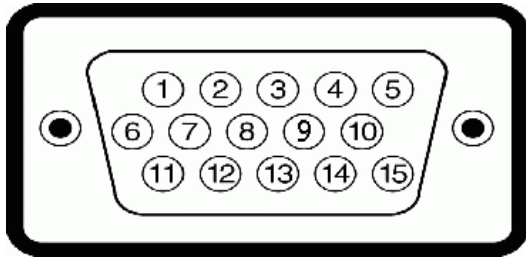
Numéro de Côté Moniteur du câble signaux 15 broche
