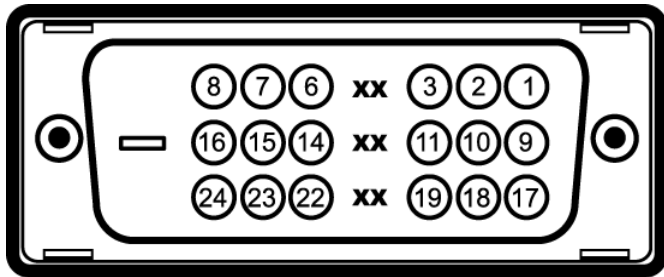
Numéro de Côté Moniteur du câble signaux 24 broches
